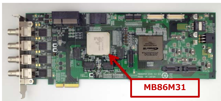
写真2 評価ボード MB86M31-EVB
