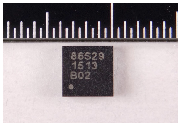
写真 1 : MB86S29 カメラフロントエンジン
