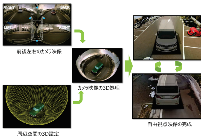
図1 全周囲立体モニタシステム ( クリックで拡大 )
