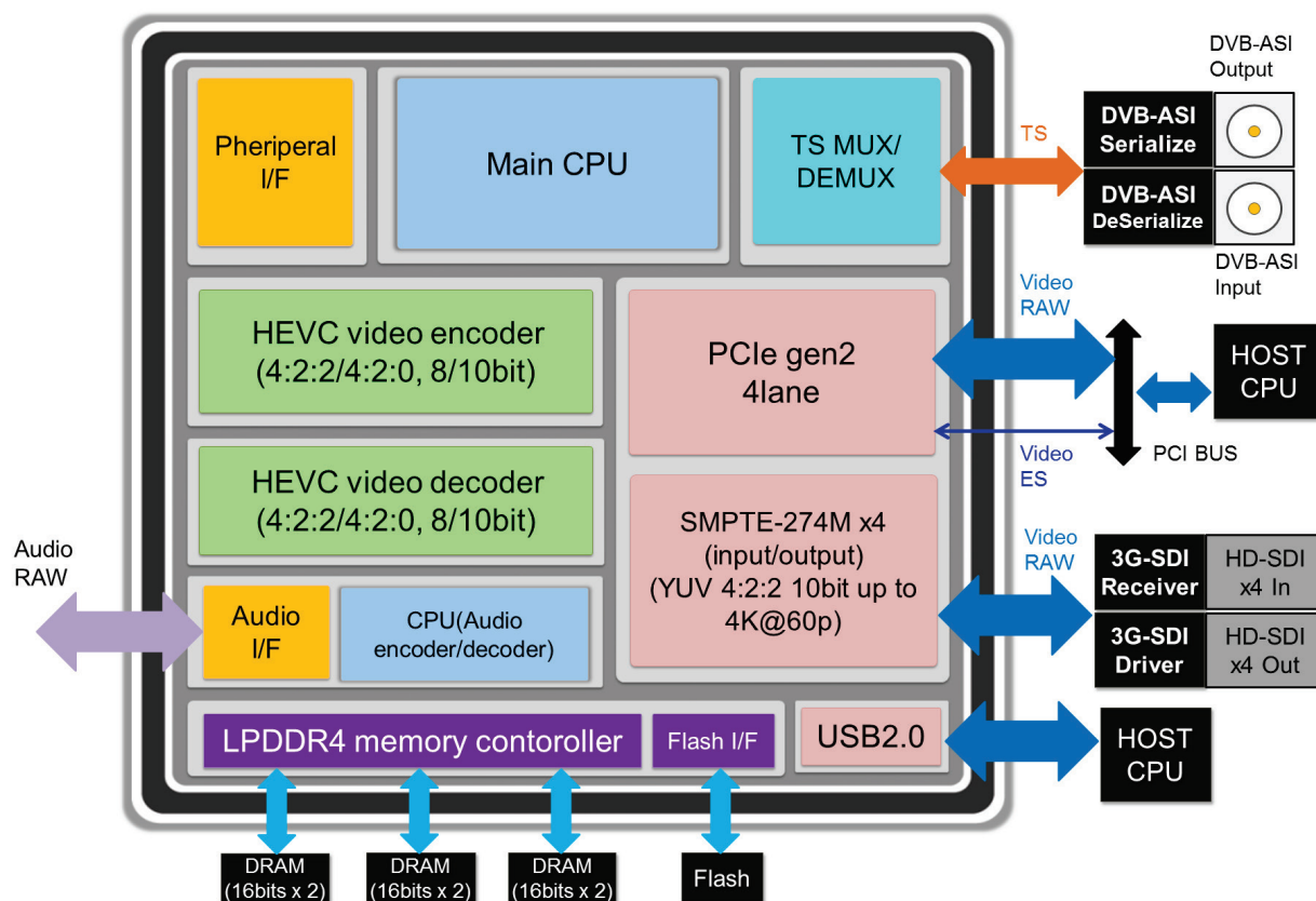
図：SC2M50 ブロックダイヤグラム ( クリックで拡大 )
