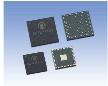
写真：SC1220 シリーズ 外観
